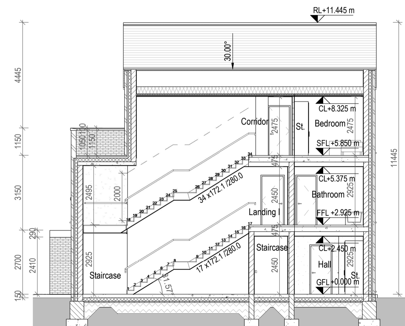
5 Section A-A 1 : 100
